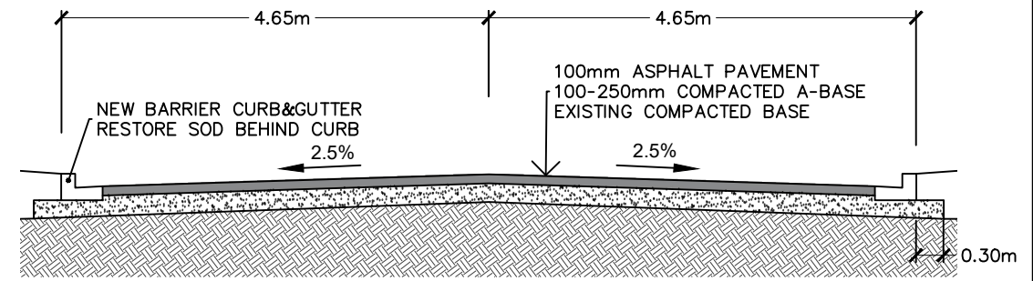
CROSS SECTION STA 0+005 SCALE: 1:75
